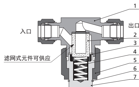
图示为烧结式 FT 系列过滤器
