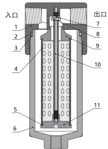
图示为滤网式 FH 系列过滤器
