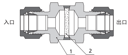
图示为烧结式 FW 系列过滤器
