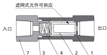
图示为烧结式 FI 系列过滤器
