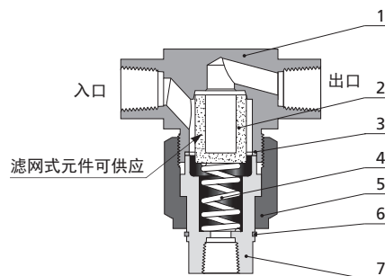
图示为烧结式 FB 系列过滤器
