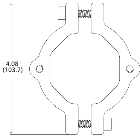
卡箍视图
