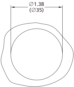
面板安装固定开孔
