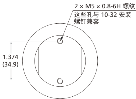
底部安装螺丝孔
