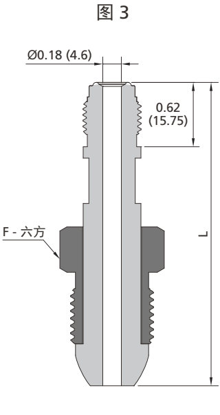
面密封阳螺纹 (FR)
