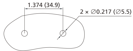
底部安装固定开孔
