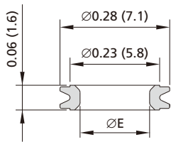
C 形垫片标准型
