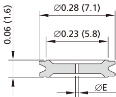
C 形垫片限流型 (仅限 CS11)
