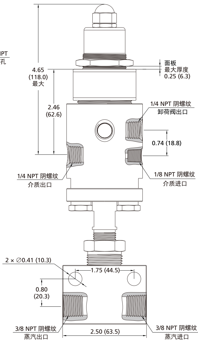
面板安装固定开口
