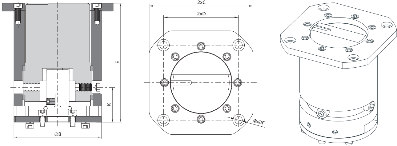
底部安装孔
