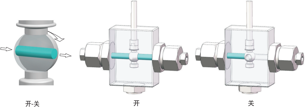
三通结构
