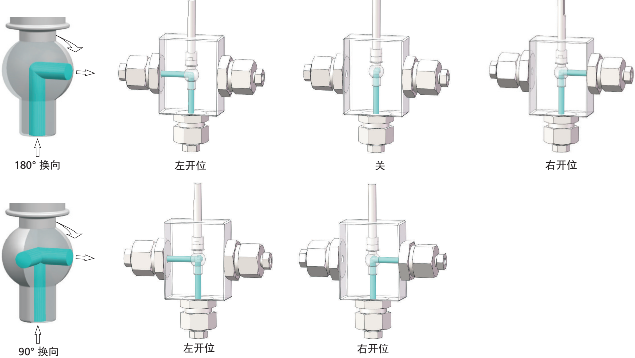
三通结构
